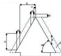
TELHADO A 60°
