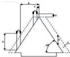
TETTO A 60°
