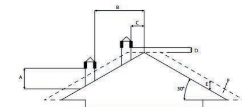
TETTO A 30°
