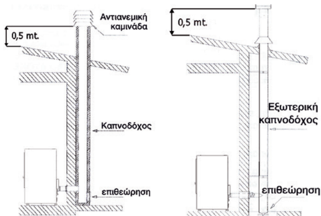
Εικ. 2: σύνδεση στην καπνοδόχο
