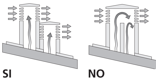
Fig. 5: características de la tapa de la chimenea
