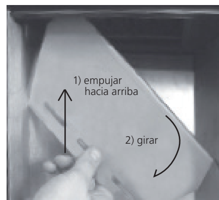
Fig. 17: extracción de la placa cortafuego
