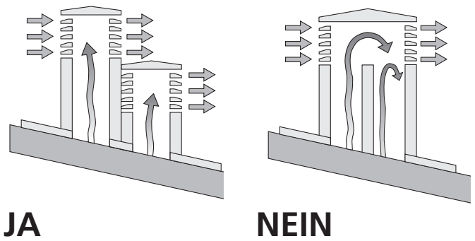
Abb. 5. Eigenschaften des Schornsteins
