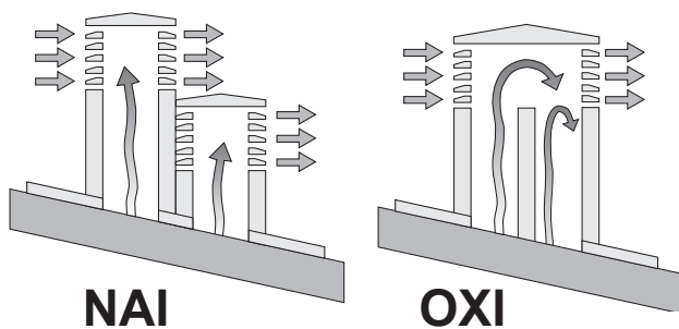
Εικ. 5: χαρακτηριστικά της απόληξης καπνοδόχου
