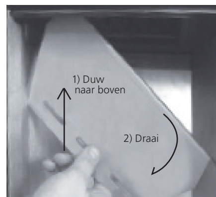
Afb. 17: verwijdering van de vlamplaat
