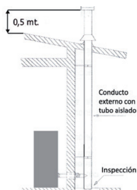
Fig. 3: conexión a un conducto externo con tubo aislado o doble pared y cumbre antiviento
