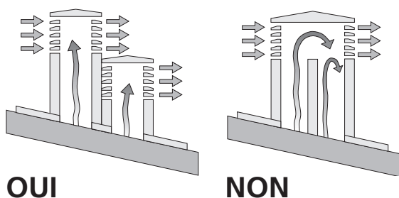
Fig. 2: caractéristiques de la cheminée
