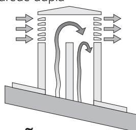
Fig. 3: ligação a um tubo externo com tubo isolado ou parede dupla
