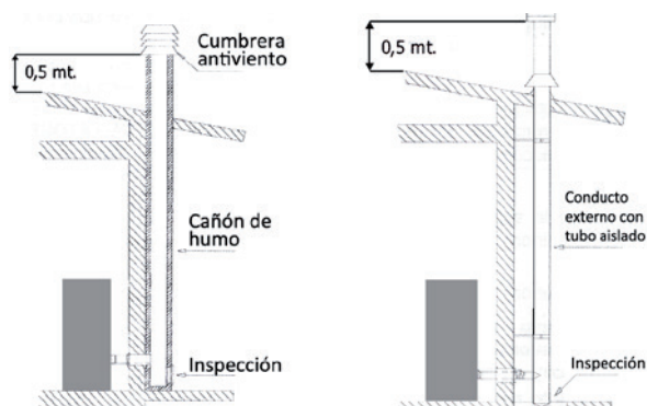
Fig. 2: conexión con el cañón de humo
