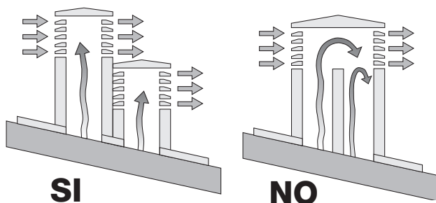
Fig. 5: caratteristiche del comignolo
